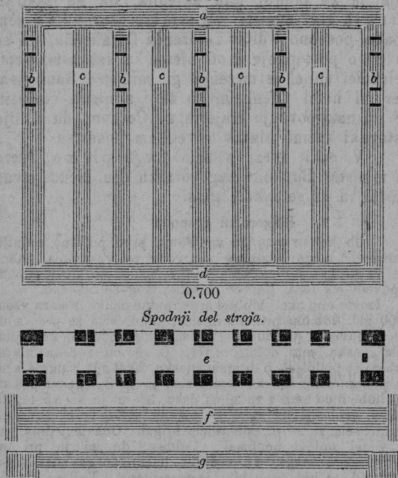
Stroj za pletenje ležakov in stojakov.
