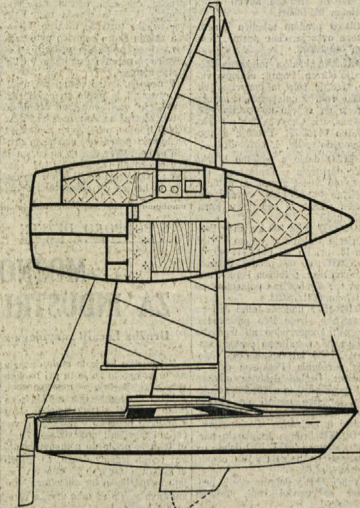
«Comet 700» — osnovni podatki: dolžina 7 metrov, maksimalna širina 2,49 metra, višina glavne kajute od 1,54 do 1,90 metra, ugrez od 0,65 do 1,8 metra, izvir 1.100 kilogramov, BRT pod 3 tone, gradbeni material ojačane poliesterske smole. Jadra: glavno jedro 9,70 kvadratnega metra, gena 17,70 ali 14,50 kvadratnega metra, flog 10,80 kvadratnega metra, nevitno jadro 5 kvadratnih metrov, spinaker pa 41,80 metra.
