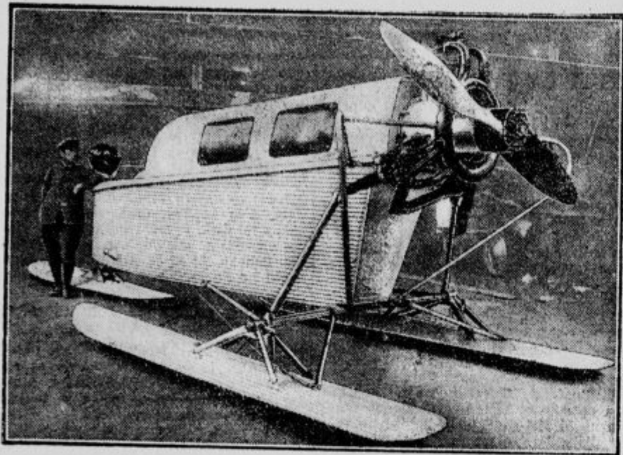
Ruske zračne »smuči«, ki dosežejo s pomočjo letalskega propelerja hitrost 120 km na uro. Aparat je razstavljen na mednarodni razstavi »Ilac« v Berlinu.
