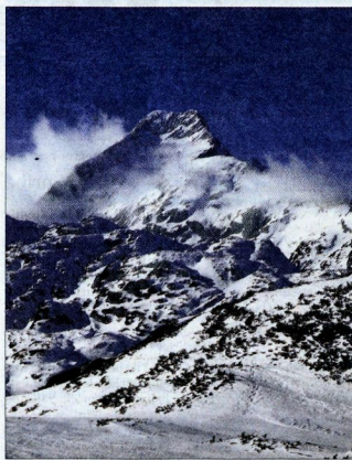
Pogled na Ojstrico z Deske.
