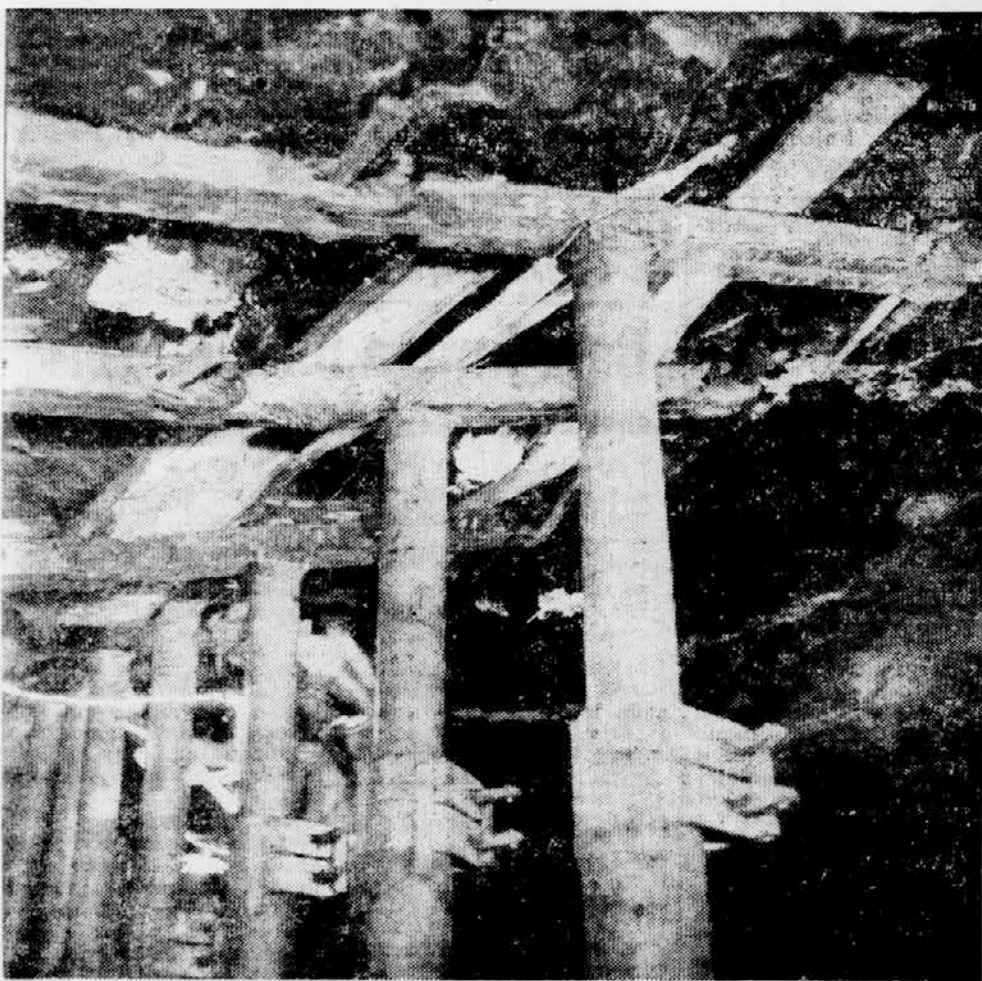
JAMSKÉ STOKÉ TIPA »VALENT«, IZDELEK STT
