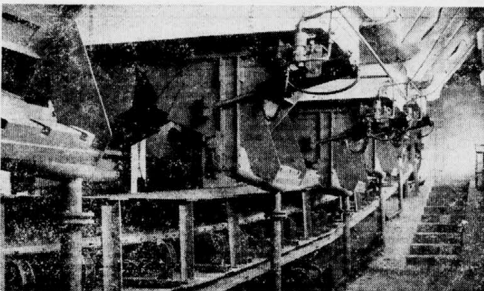
DEL MECHANIZACIJE OPREME, SEPARACIJA IBARSKI RUDNIK, KI JO JE IZDELALO IN OPREMILO PODJETJE STT TRBOVLJE
