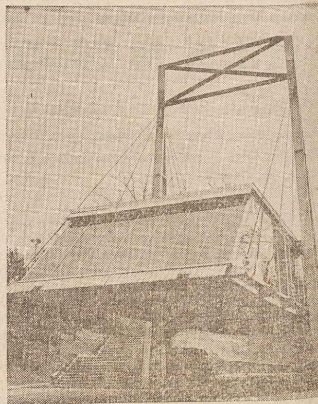
DREVESNI DOM — Na Mednarodni razstavi domov v Turinu v Italiji je bila razstavljena tudi "drevesna hiša" arhitekta Lorenza Papi-ja iz Florence. Izdelana pretežno iz jekla in stekla, visi na jeklenih kablích na dveh močnih opornikih.
