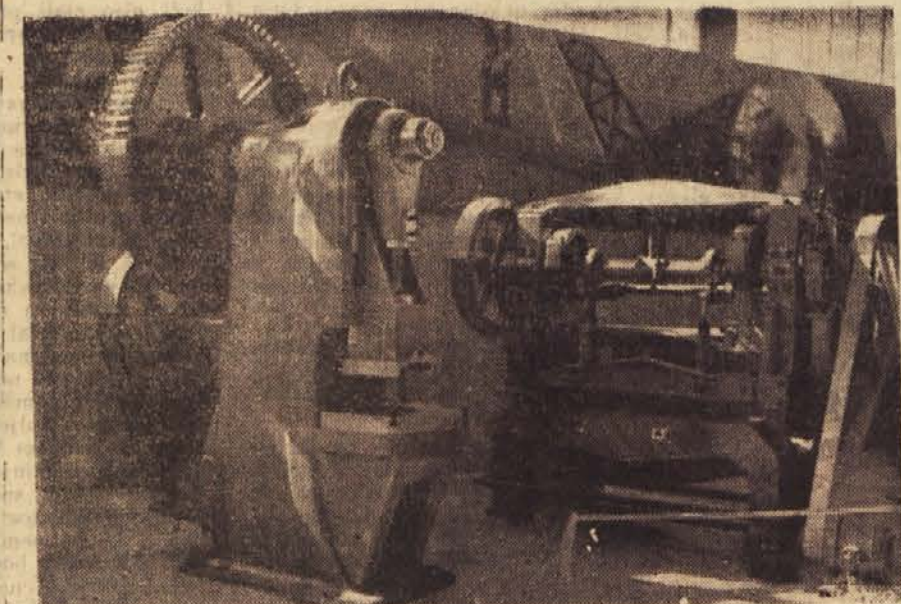
Mehanične stiskalnice — proizvod tovarne »Ivo Lola Ribar« v Železniku
