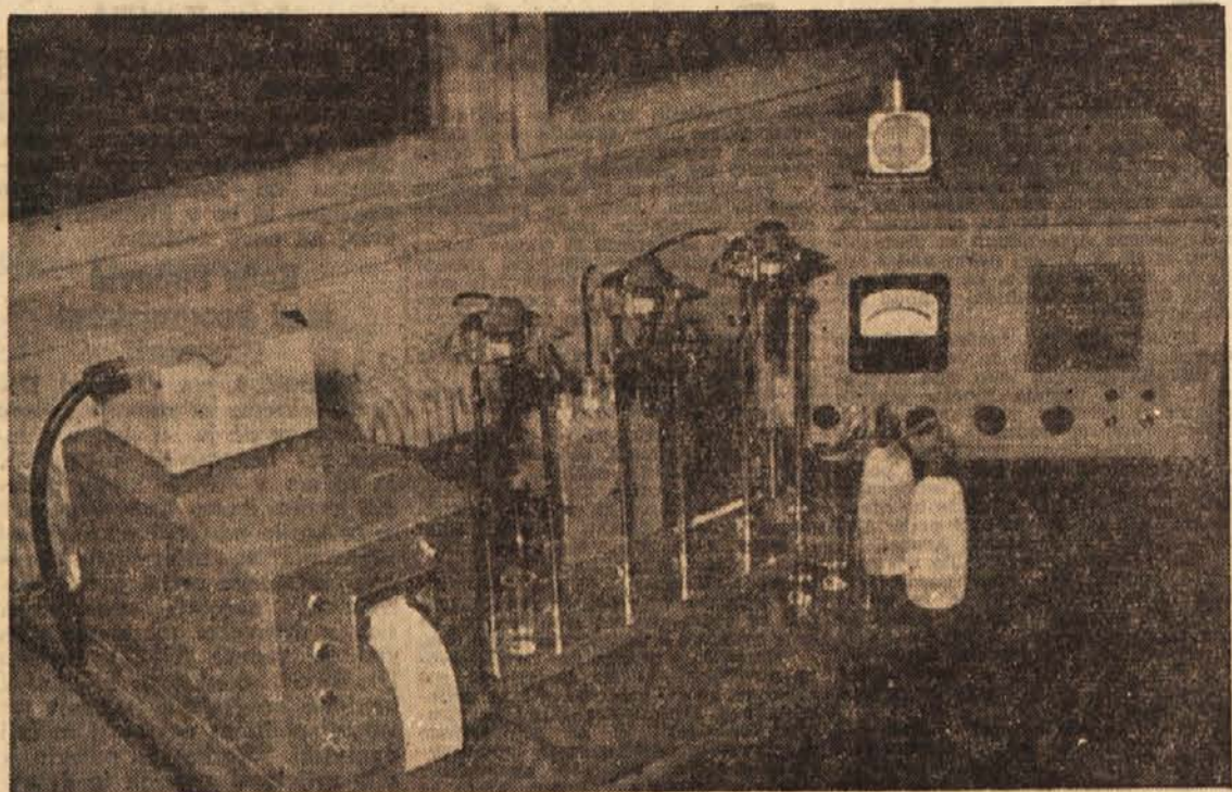
Priprave za merjenje radioaktivnosti v raztopinah
