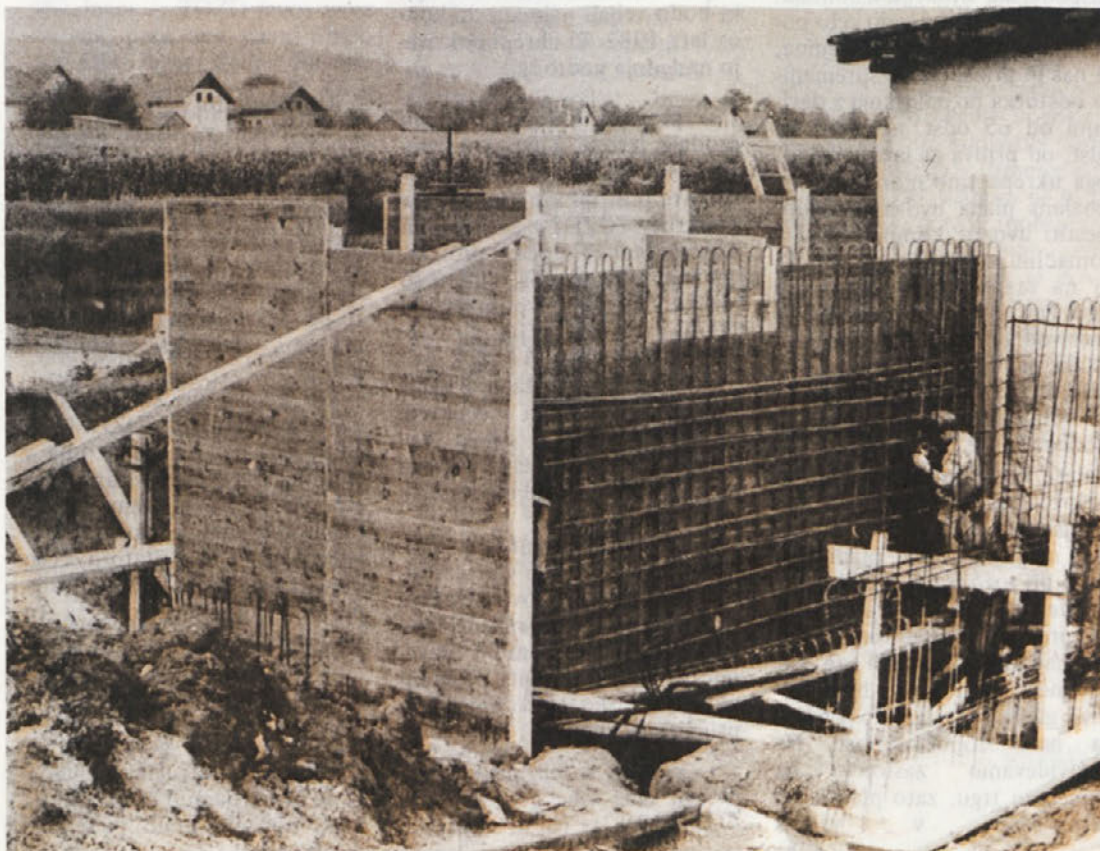
Pogled na gradbišče črpališča tehnološke vode v Straži, ki bo zgrajeno že čez dva meseca.
