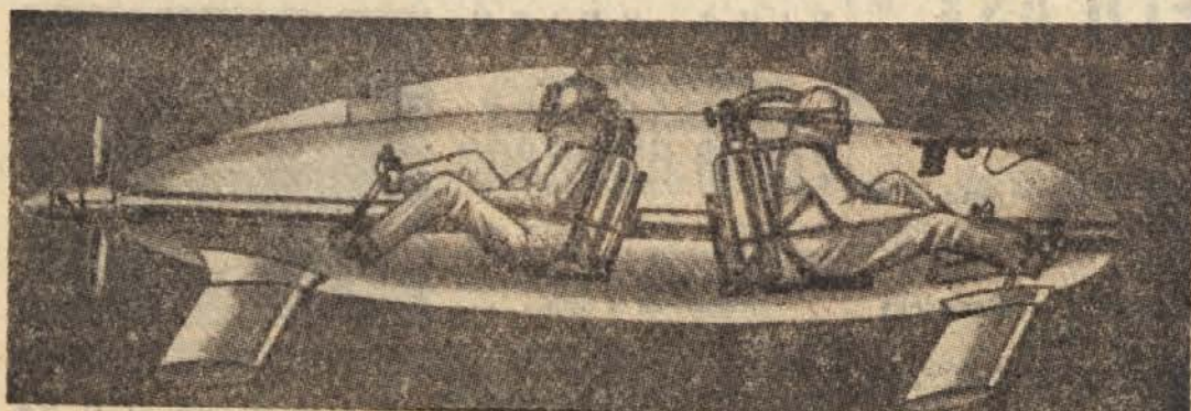
»Minisub« je dolg 4,37, širok 0,56, visok 1,07 m, tehta pa 177 kg
