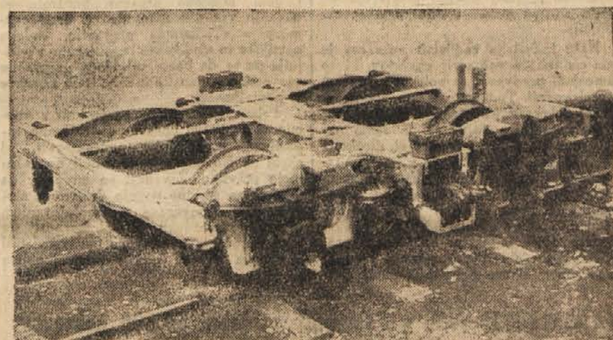
Podstavni voziček štiroosnega ozkotirnega jeklenega vagona I. in II. razreda, izdelanega v glavni železniški delavnici v Sarajevu. Pred vojno takih vagonov v Jugoslaviji niso izdelovali
