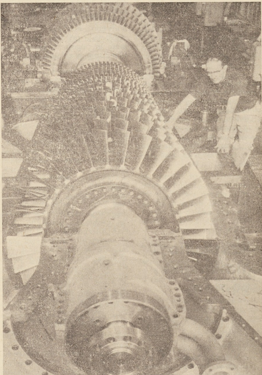
Rotor plinske turbine, plinsko-parne elektrarne DO TET. V ospredju je 18 stopenj kompresorskega dela, v sredini gorilniški del rotorja, na zadnjem delu rotorja so tri stopnje lopatic plinske turbine. Teža je 16 ton, dolžina 8 m in premer 2,3 m.
