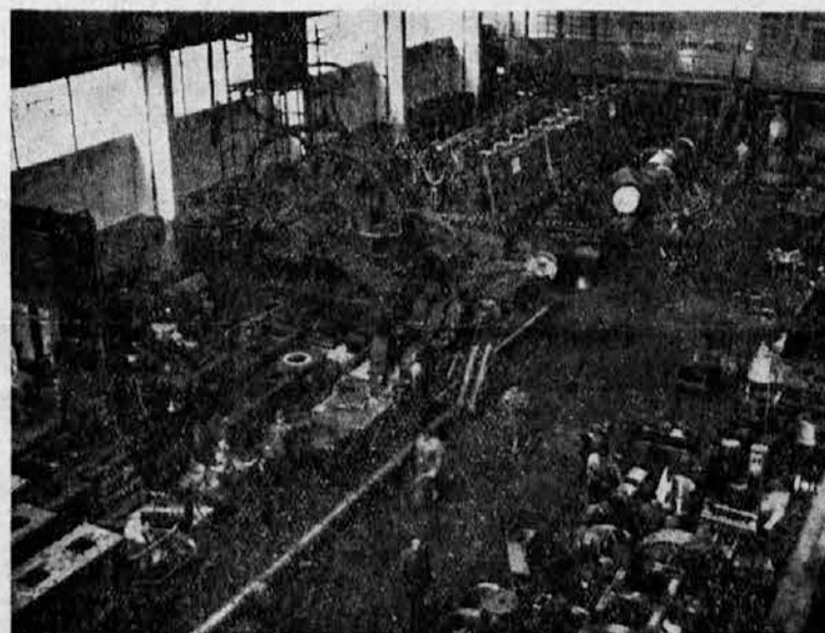
Tovarna strojev Sv. Andreja gradi izvrstne ladijske stroje. Slika nam kaže montažo Dieslovega stroja za norveško ladjo.
