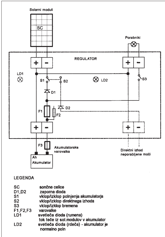
Slika št. 5: Regulacija polnjenja akumulatorja za enojni solarni sistem
