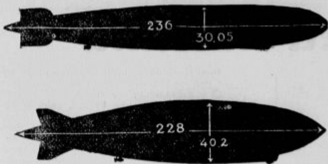
Novi »Zeppelin«. V Friedrichshafnu so začeli graditi nov zrakoplov »Zeppelin« novega tipa (spodaj), ki bo nekoliko krajši, zato pa znatno večjega premera nego sedanji »Groß Zeppelin« (zgoraj) in bo nosil ime »LZ. 120«. Novi zrakoplov bo dolg 228 metrov premer pa bo znašal na najširšem mestu približno 41.2 m. Zato bo tudi prostornina novega zrakoplova skoraj za polovico večja nego jo ima sedanji »Zeppelin«, to se pravi 200.000 kub. metrov proti 105.000. Štirje Dieslovi motorji novega zrakoplova bodo mogli razvijati 3600 k. s. proti 2650 k. s. sedanjega »Zeppelina«.
