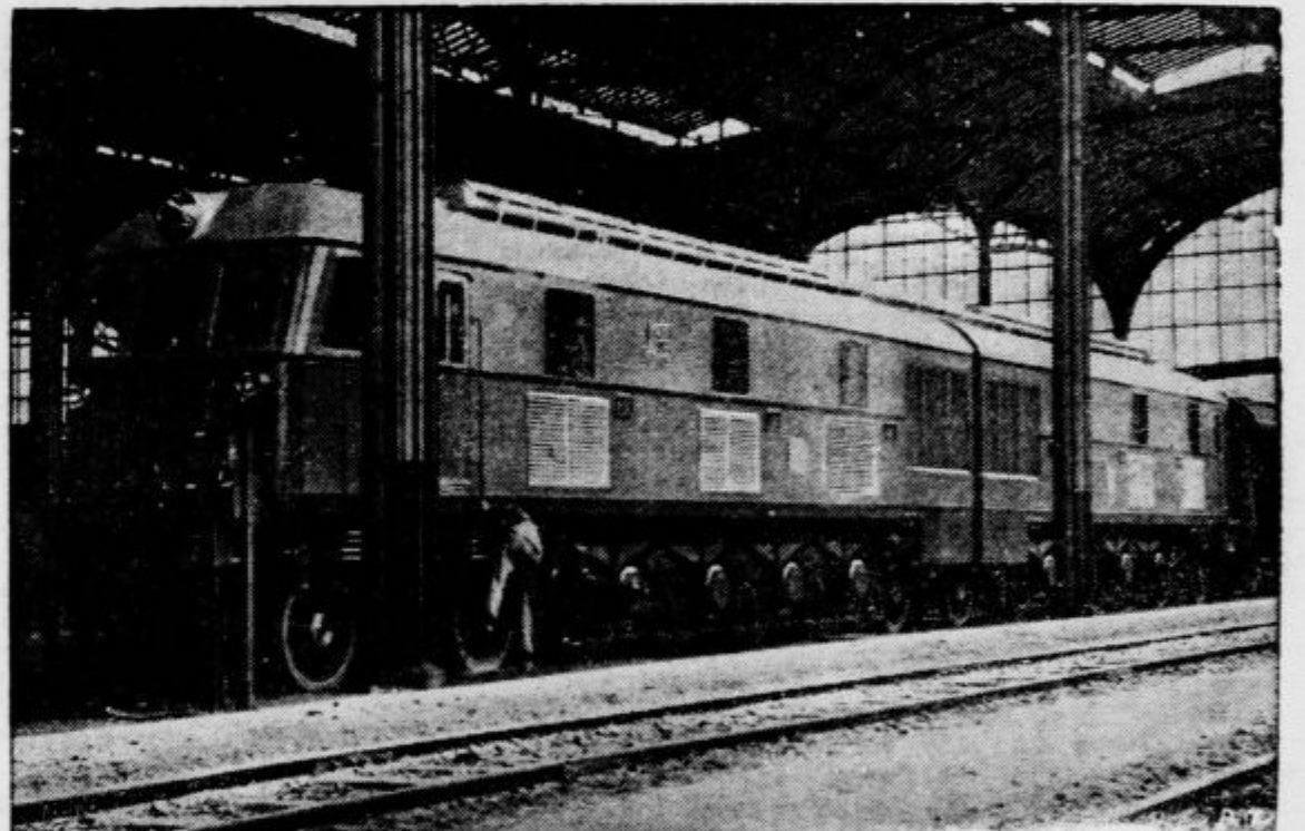
V Švicci so zgradili za rumunske državne železnice lokomotivo, ki meri v dolžino 29 m in tehta 234 ton. Poganjajo jo Dieslovji motorji s 4400 ks
