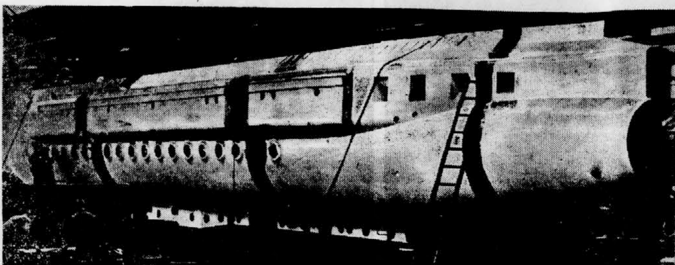
KMALU NA IZLET — Trup prve turistične podmornice je že skoraj povsem izdelan. Na vrhu so tanki, ki jih bo napolnila voda, kadar se bo hotel mezoskaf potopiti v globine.
