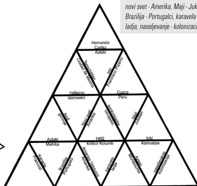
Slika 4: Rešitev igre tromino
