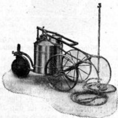
Pod. 3. Vozna škropilnica „Freya“ na 3 kolesih.
