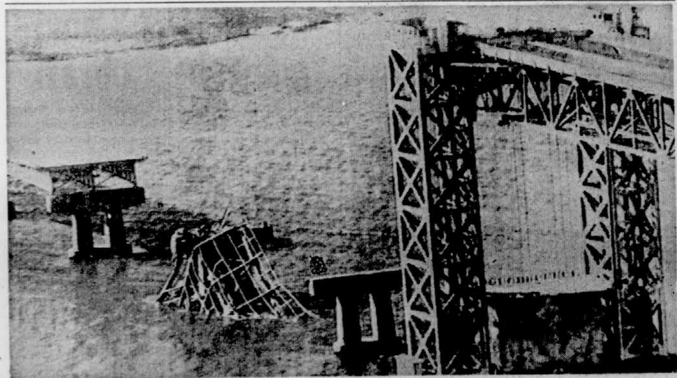
MOST SE JE VDAL — Vse kaže, da so se graditelji mostu Sidney Lanier čez reko Brunswick v ameriški državi Georgia uračunali: ko je čezenj zapejal težko natovorjen vlak, se je del 1600 metrov dolge konstrukcije sesedel. Človeških žrtev na srečo ni bilo.
