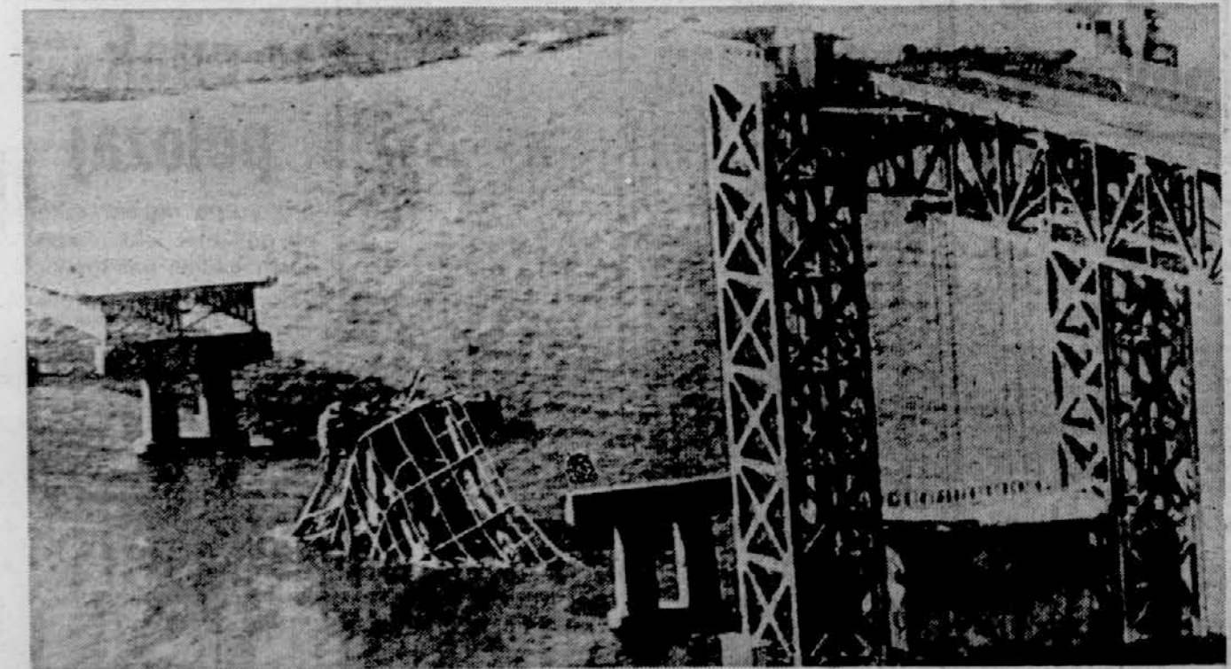
MOST SE JE VDAL — Vse kaže, da so se graditelji mostu Sidney Lanier čez reko Brunswick v ameriški državi Georgia uračunali: ko je čezenj zapeljal težko natovorjen vlak, se je del 1600 metrov dolge konstrukcije sesedel. Človeških žrtev na srečo ni bilo. Telefot: UPI
