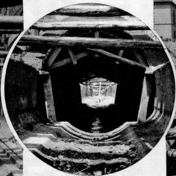
Razne gradbene faze pri gradbi kanala za Počehovski potok v Mariboru
