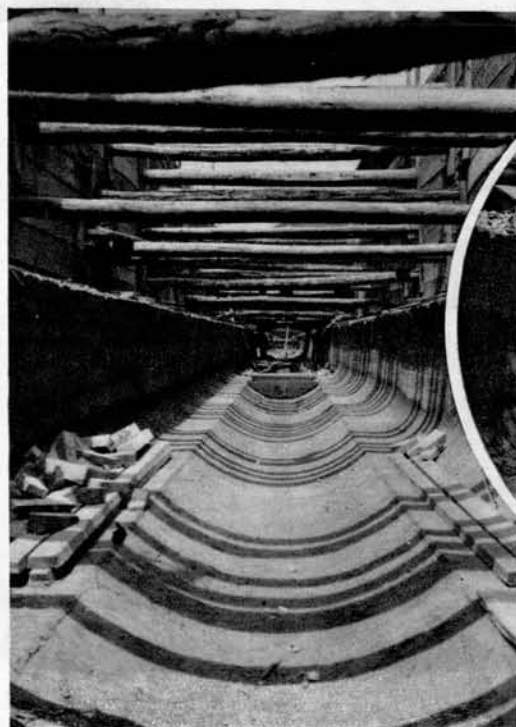
Razne gradbene faze pri gradbi kanala za Počehovski potok v Mariboru
