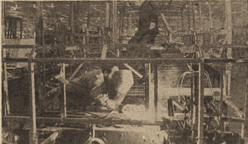
Od surovin do izdelanega avtobusa preteče v Avtomontaži 17 dni. Delov in dela je namreč zelo veliko
