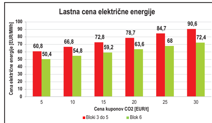
Diagram 2: grafični prikaz primerjave povprečne lastne cene električne energije med obstoječimi bloki 3-5 in blokom 6 glede na ceno CO 2 (za celotno obratovalno obdobje) in prodajno ceno
