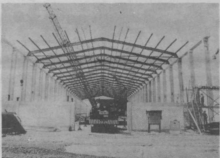
Ena najvažnejših industrijskih gradenj v Sloveniji je tovarna sladkorja v Ormožu. Glavni graditelj je GRADIS. (Foto arhiv Gradisa)
