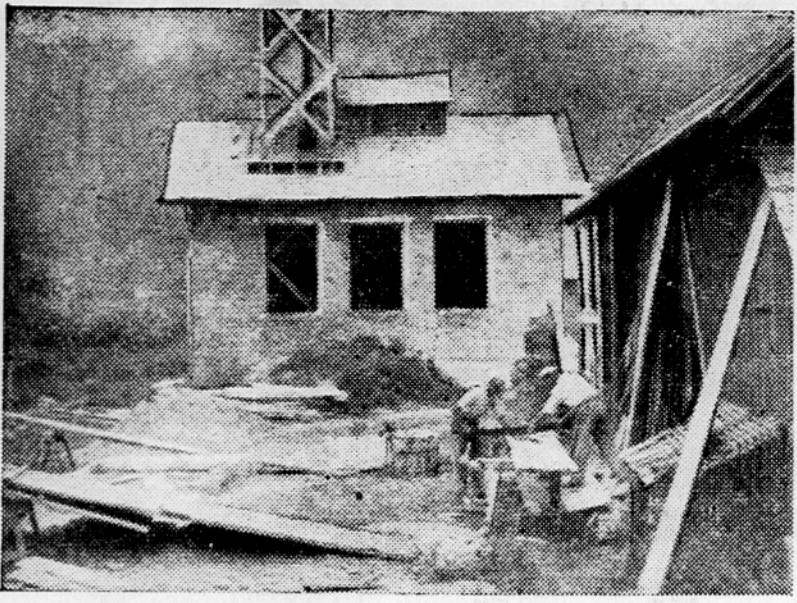
Zadruga v Češnjici gradi sušilnico lesa in strojno, kjer bodo montirali parni kotel. Para bo služila za sušenje lesa in za pogon generatorja.
