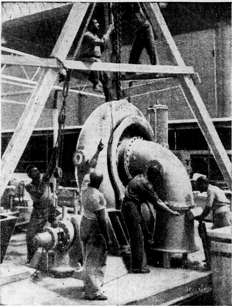
Na veleselju v Smirni postavljajo Litostrojevo turbino, izdelano za hidro- centralo Zavrčje pri Dubrovniku
