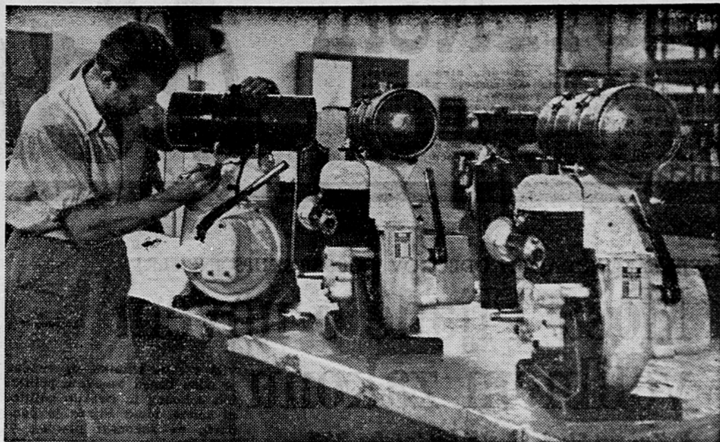
Montaža bencinskih motorjev v končni fazi
