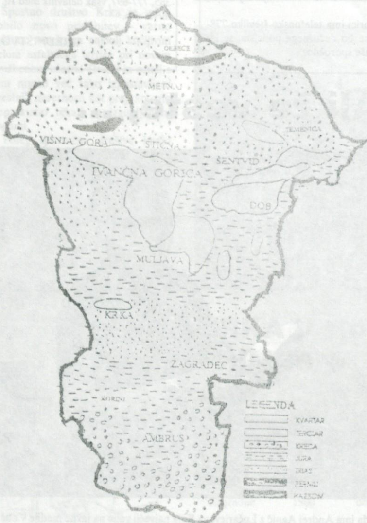
Poenostavljena geološka karta našega ozemlja.
