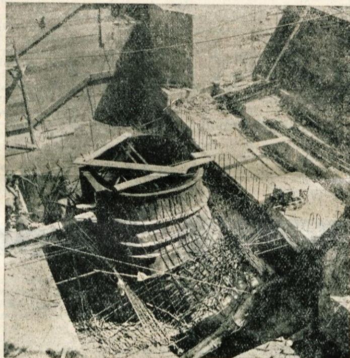
Silka prikazuje jekleno oblogo in armaturo za sesalno cev. Nad njo so kasneje zabetonirali špiro in montirali turbino
