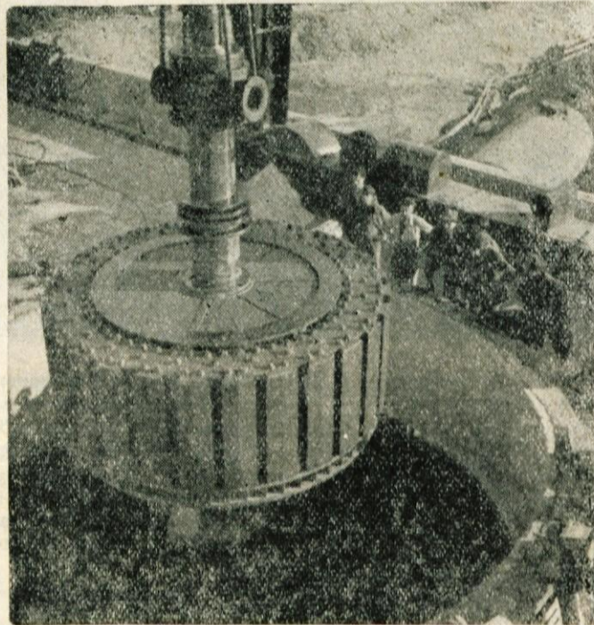
100 tonski maček glavnega portalnega žerjava, ki je viden na sliki 3, spušča v montažnico rotor, težak 65 ton
