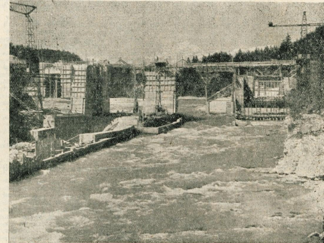
Najprej so začeli graditi desno polovico elektrarne. V ta namen so zgradili betonske pregrade, s katerimi so vodo speljali v levi del korita.
