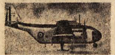
»Breguet 940 - Intégral«, na katerem vzbujajo pozornost veliki propelerji. Pogonjajo jih 4 plinske turbine po 360/400 KS. Tudi na zunanji je videti, da se to letalo po konstrukciji znatno razlikuje od običajnih potniških letal.
