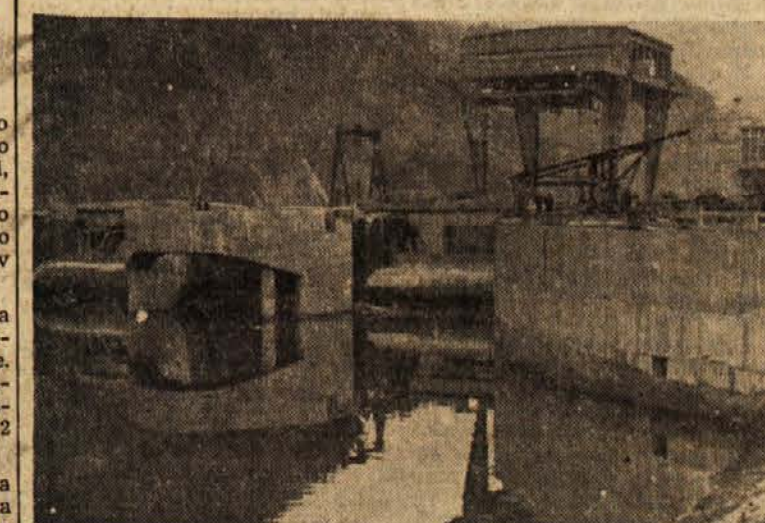
Pogled na del hidroelektrarne v Vuhredu z vtočnim objektom prvega turbinskega stebra in velikim portalnim žerjavom
