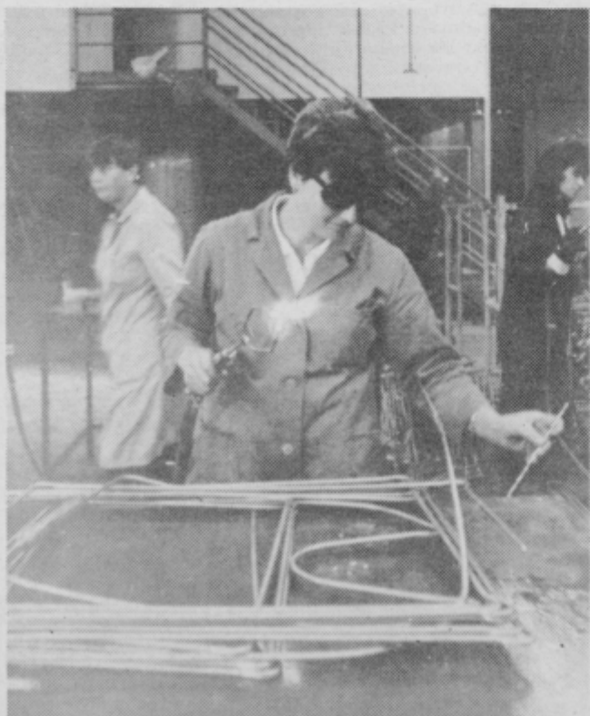
Nada Artič, delavka Gorenjevega tozda v Rogatcu, ki se je dobro usposobila za delo pri varjenju cevni izparilcev s povratno cevjo, kapilarno in tipalom termostata, kar je novost v proizvodnji tozda Kondenzatorji
