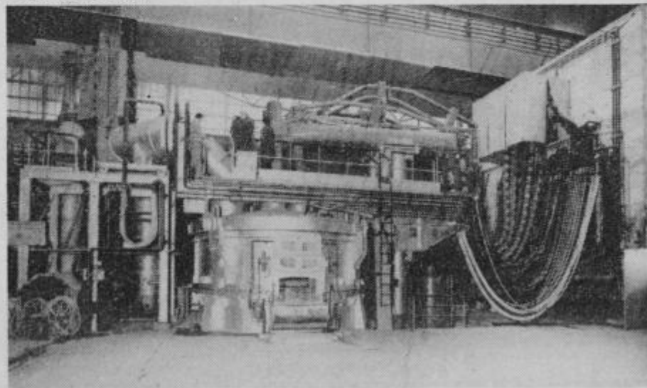
Zadnja jeklarska pridobitev: nova 50-tonska elektroobložna peč
