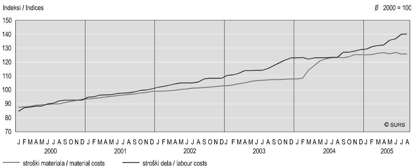
Slika 3: Indeksi gradbenih stroškov, Slovenija, januar 2000 - avgust 2005
