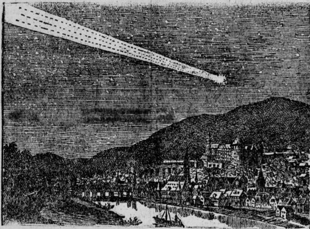
Veliki komet nad Heidelbergom leta 1618. (Po starem bakrorezu.)
