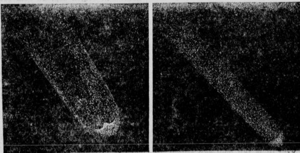
Halleyev komet ob svojem zadnjem pojavu leta 1836.
