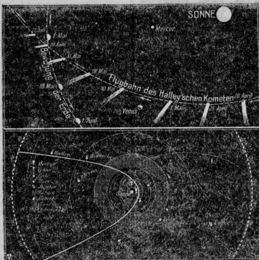
Tek Halleyevega kometa in gibanje naše zemlje.
