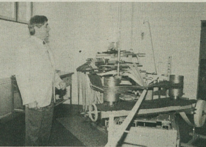
PAPIR NAMESTO PLASTIKE - Stroj, ki ga je skonstruiral Janez Habič (na sliki), vodilni strokovnjak za proizvodnjo spiralno navitih cevi v Sloveniji, bo navil 16 metrov cevi na minuto. Podjetje Spektri računa na trend proizvodnje naravi prijaznih izdelkov. (Foto: B. D.-G.)
