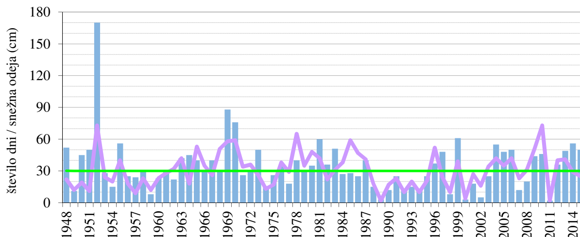
Slika 10. Letno število dni s snežno odejo (krivulja) in referenčno povprečje (zelená črta) ter najvišja snežna odeja (stolpci) v obdobju 1948–2015 v Podbrdu
