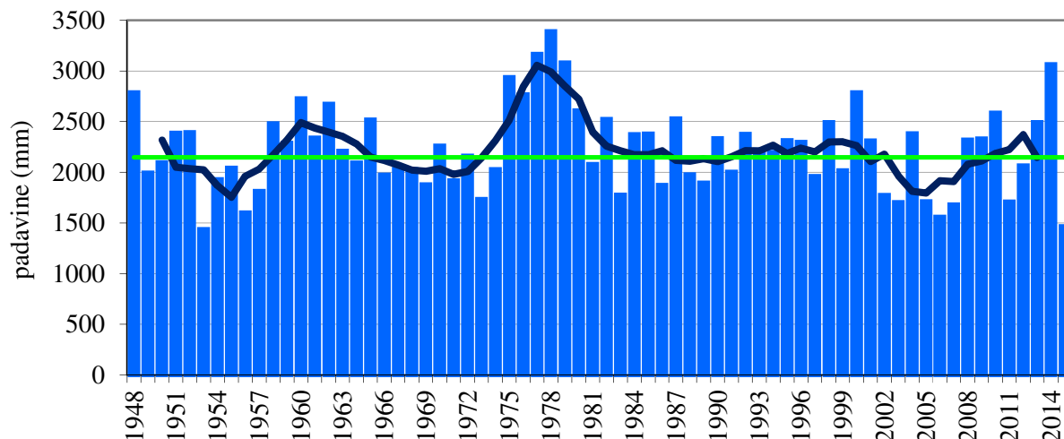
Slika 2. Letna višina padavin (stolpci) in petletno drseče povprečje (krivulja) v obdobju 1948–2015 ter referenčno povprečje (zelena črta) v Podbrdu Figure 2. Annual precipitation (columns) and five-year moving average (curve) in 1948–2015 and mean reference value (green line) in Podbrdo
