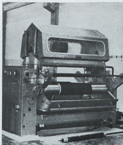
Breznapetostni jigger za barvanje blaga. Kupljen 1975
