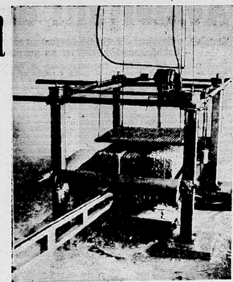
Polnojarmenik za rezanje kamna izdelek Gorških strojnih tovarn in livarn
