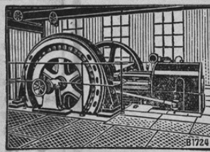
LANZOVE vročeparne Lokomobile z naravnost vezano Dynamo.
