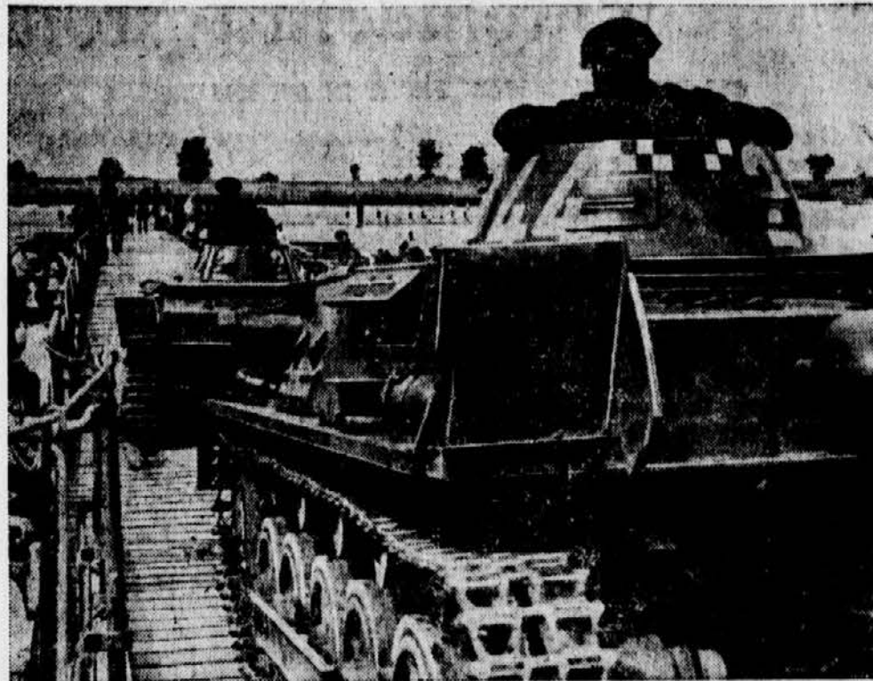
Bei einer Übung deutscher Pioniere wurde die Geschwindigkeit geprüft, mit der schwere Militärfahrzeuge, wie Panzerkampfwagen und Zugmaschinen, über eine geschlagene Brücke fahren können. Unser Bild zeigt den Augenblick, in dem Panzerkampfwagen zunächst langsam anrollen, wobei festgestellt wird, wieviel Strich die Pontons der Fähre ins Wasser gedrückt werden. (Scherl-Bilderdienst-M.)
