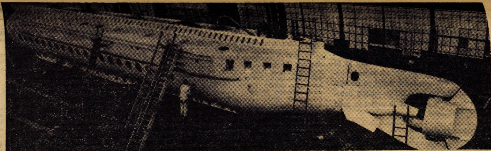
Po šestih mesecih so v Montjeyju v Švici zgradili podmornico, ki bo služila za podvodno izletništvo. Na sliki vidimo 30 metrov dolgo podmornico, ki je zdaj dokončana. Podmornico pa morajo še notranje opremiti. Konstruktor je profesor Piccard.
