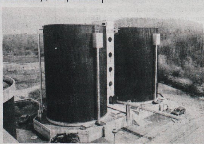
Dve gnilišči – prostornina vsakega je 1800 m 3
