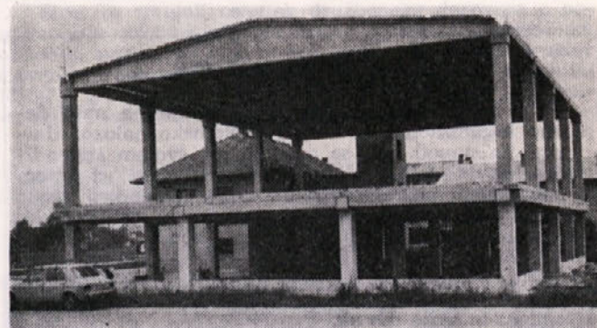
Montažna konstrukcija za Gasilski dom Ostrožno
