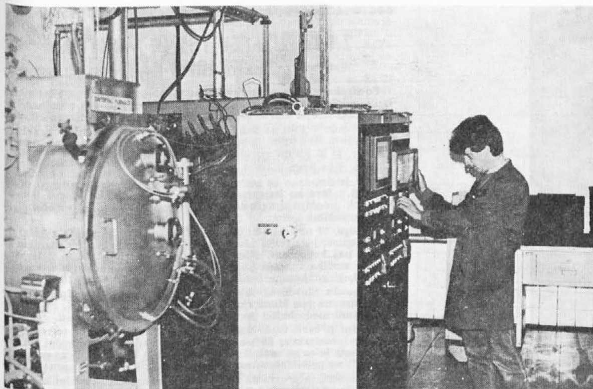
Vakuumska peč za sintranje v oddelku karbidnih trdin. Delovni proces je voden računalniško.
