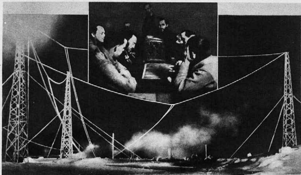
Radio na južnem tečaju.
