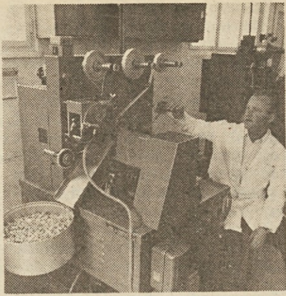
Strojno navijanje nizkonapetostnih kondenzatorjev. Pri stroju je Rudi Bizjak.
