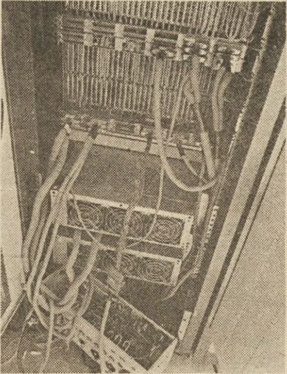
Računalnik 160, z zadnje strani, namenjen je za avtomatsko telefonsko centralo Metaconta 10 C.
