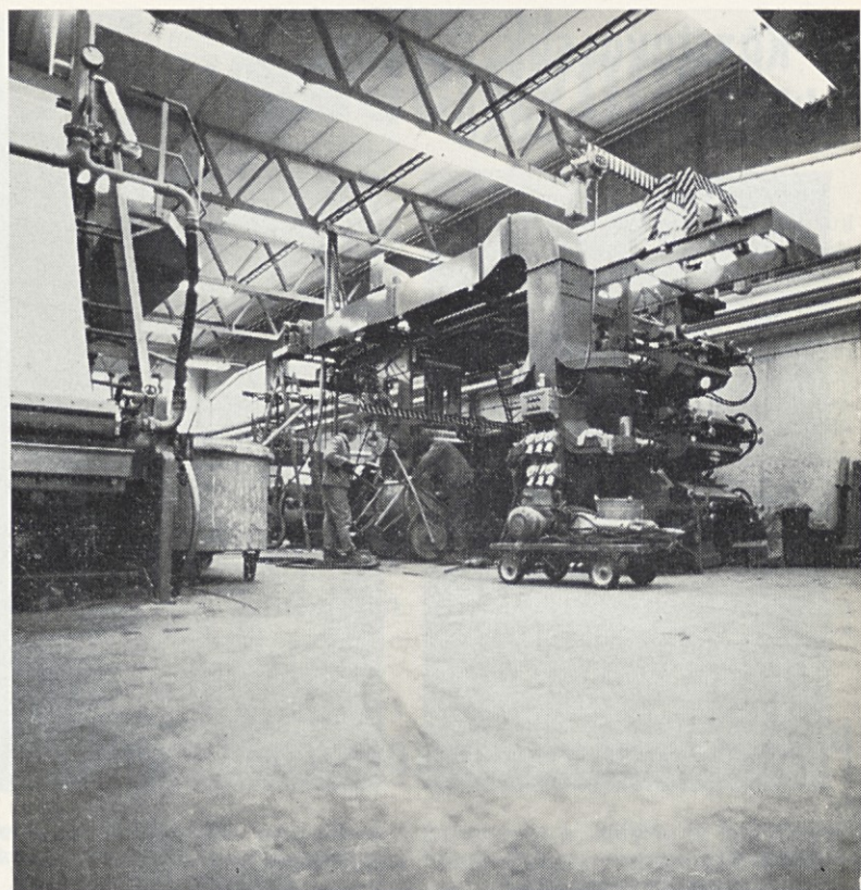
Pripravlja se zopet nekaj novega. Stroj v montaži
