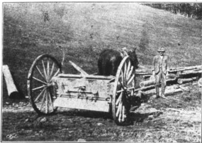
Podoba 78. (izvir) Trosilo za gnojilo tvrdke Hofherr & Schrantz, prenamerjeno za gorat svet po Weinzierlu.
