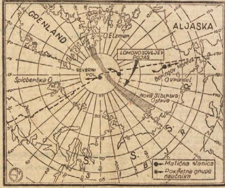
Področje Severnega tečaja
