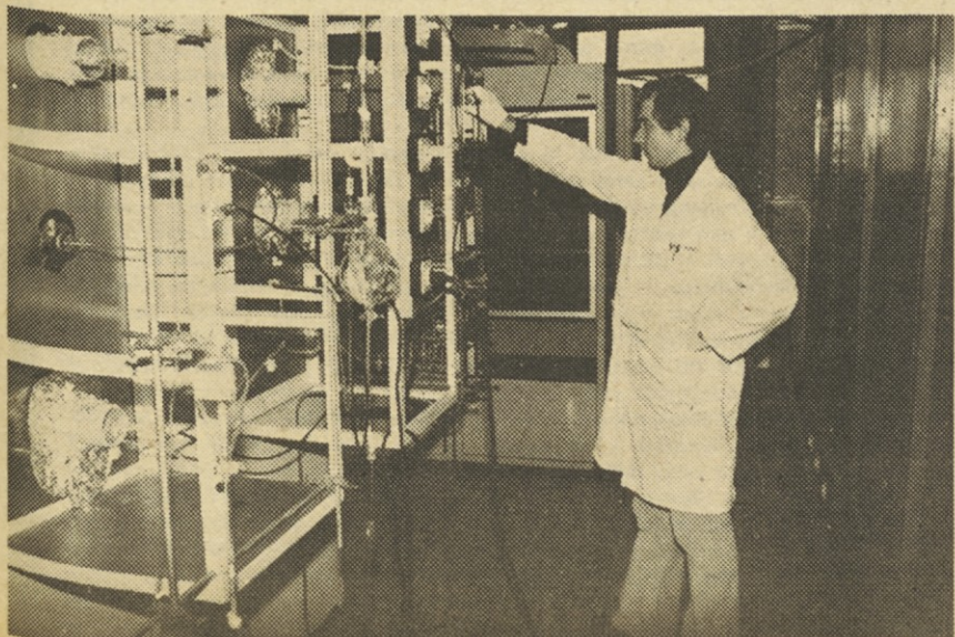
Kontrola pretoka plina v difuzijski peči — Ivan Kahne.
