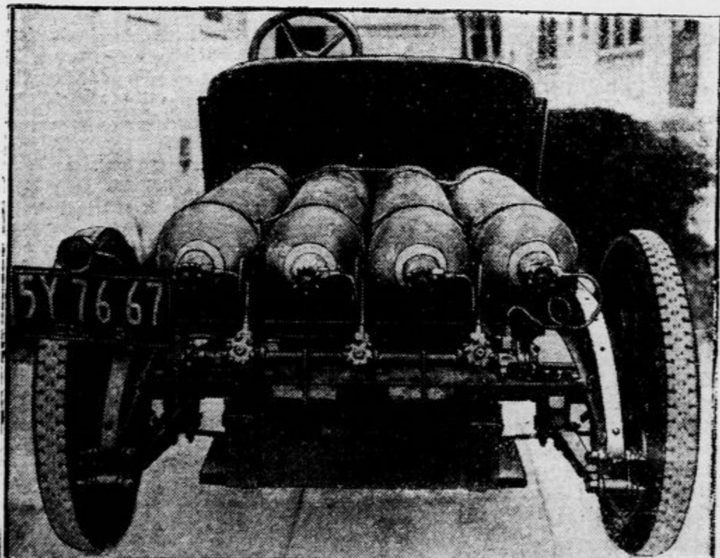
Sasija avtomobila na pogon s svetilnim plinom, ki je shranjen v podolgovatih jeklenih bombah pod visokim pritiskom.
