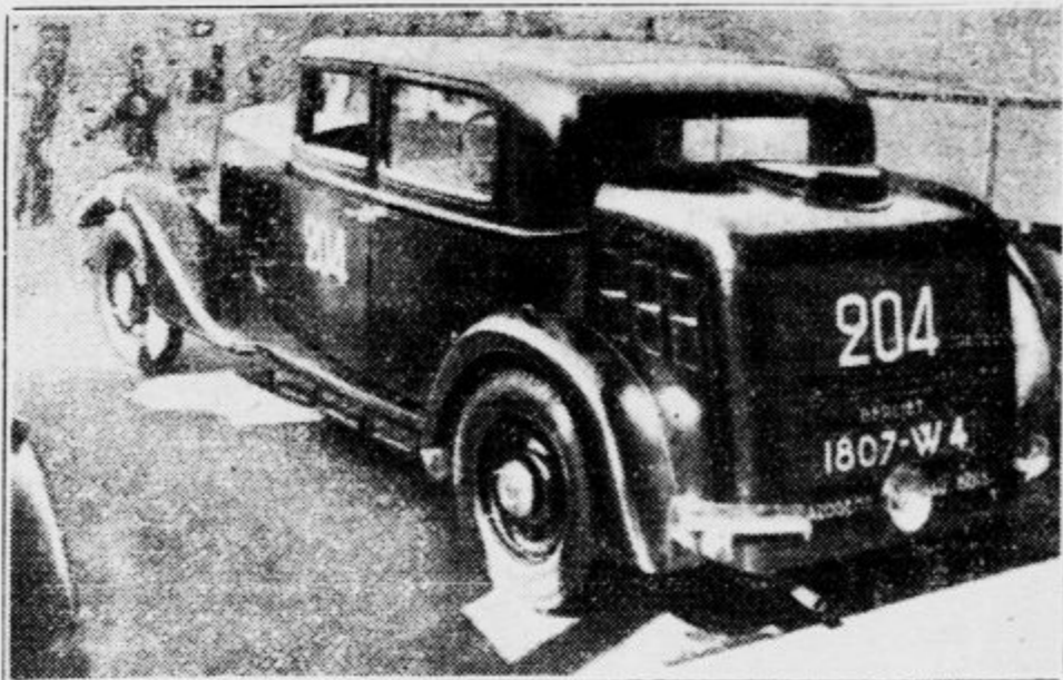
Panhardova luksuzna limuzina na pogon z ogljem. Plinski generator je montiran v nastavku na zadnjem delu voza
